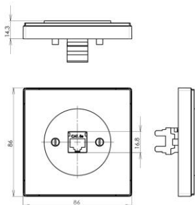
Рис 2. Розетка компьютерная, размеры
