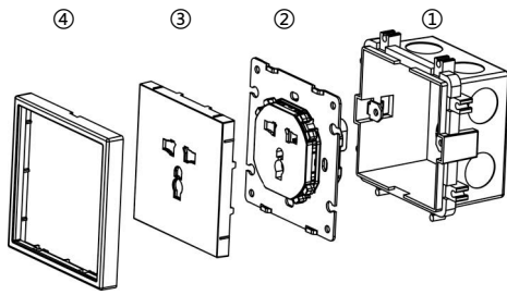
Рис 5. Установка
