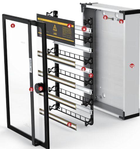
Рис.2. Распределительный щит серии Platinum intelligent с направляющими в каркасе в разборе.
