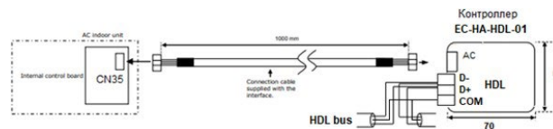
Схема подключения
