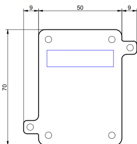
Рис. 4. Габариты – Вид сзади (мм)
