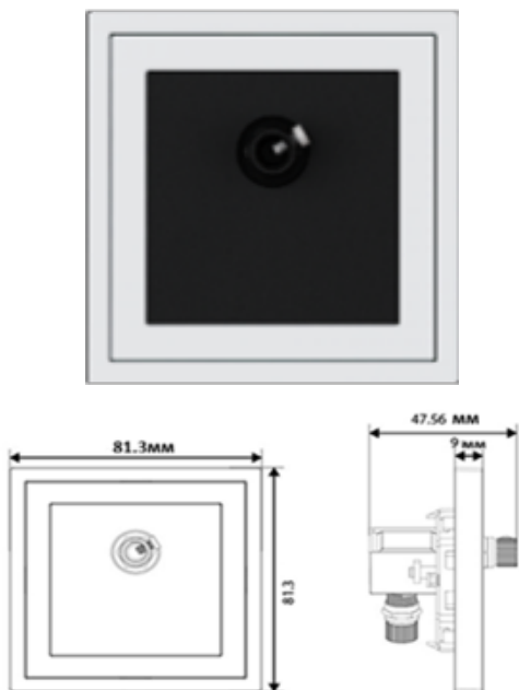
Телевизионная TV-F-Type розетка серии Xelent
