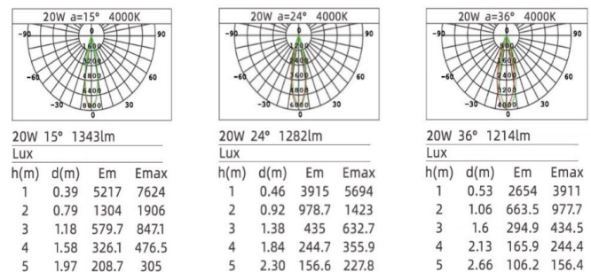
Рис. 3 — Светораспределение светильника с фиксированной цветовой температурой
