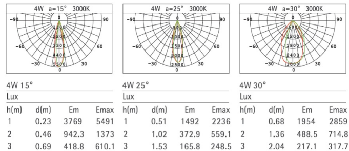
Рис. 3 — Светораспределение светильника с фиксированной цветовой температурой
