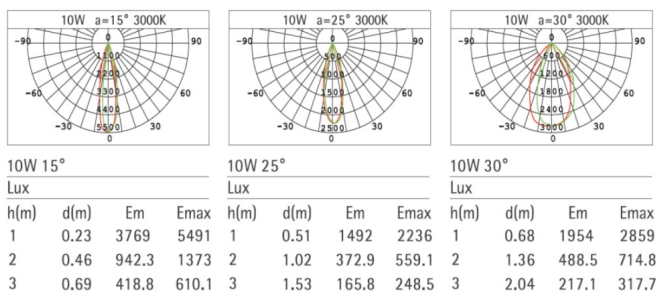
Рис. 3 — Светораспределение светильника с фиксированной цветовой температурой
