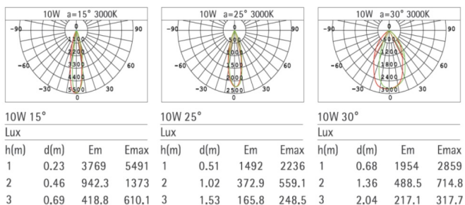
Рис. 3 — Светораспределение светильника с фиксированной цветовой температурой
