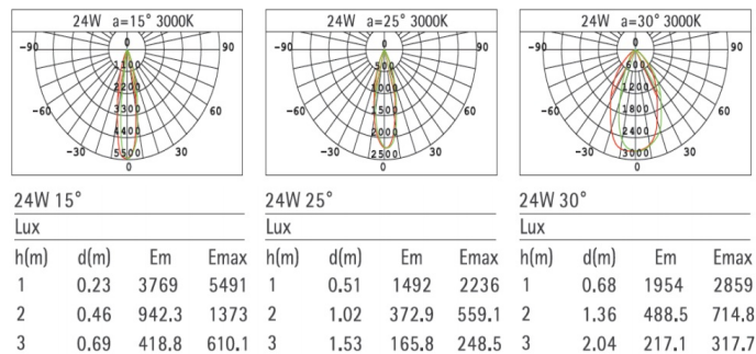
Рисунок 2 — Светильник с регулируемой цветовой температурой (ССТ) — Распределение света
