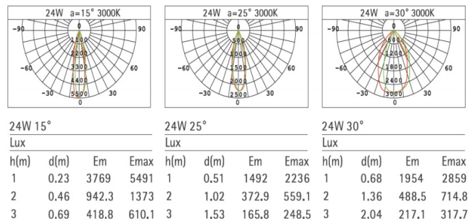
Рисунок 3 — Светильник с фиксированной цветовой температурой (ССТ) — Распределение света
