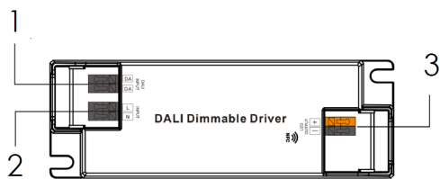
Рис.2. Основные элементы устройства
