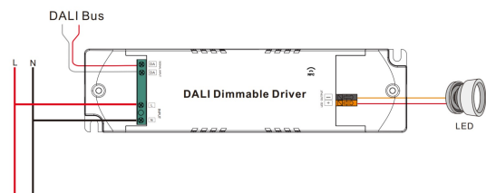
Рис.4. Схема проводки для подключения одноцветного светодиодного светильника к шине DALI
