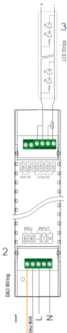
Рис.2. Основные элементы устройства
