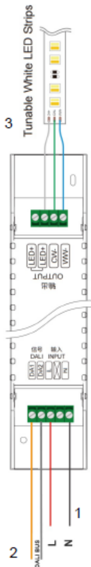
Рис.2. Основные элементы устройства
