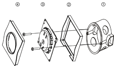
Рис. 4. Установка
