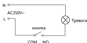
Рис 4. Подключение
