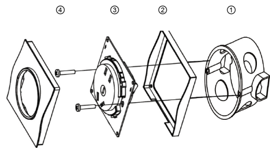
Рис. 4. Установка
