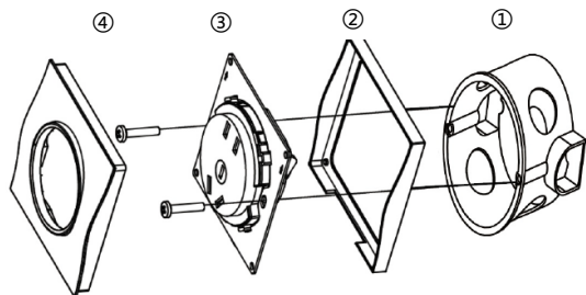
Рис 4. Установка
