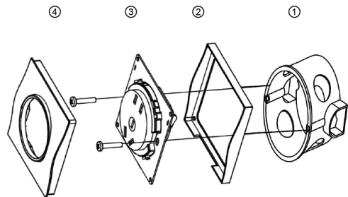
Рис. 4. Установка
