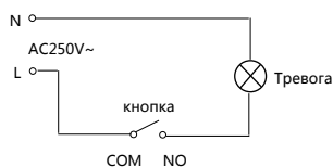
Рис 4. Подключение
