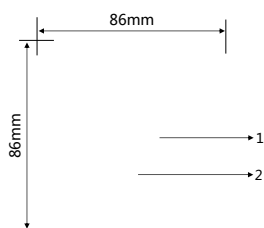
Рис 2. Размеры – Вид спереди Пластиковая рамка
