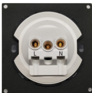
Выключатель 1-клавишный серии Eave
