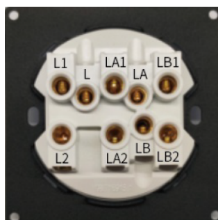
Выключатель 3-клавишный серии Eave
