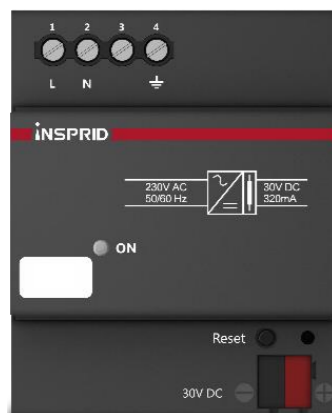
Блоки питания 320mA/640mA
